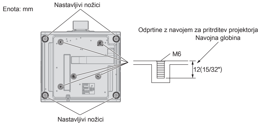
Mesta odprtin z navojem za pritrnitev projektorja in nastavljive nožice
