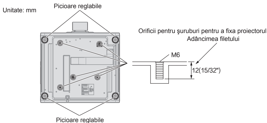
Pozițiile orificiilor pentru șuruburi pentru fixarea proiecteurului și a picioarelor reglabile
