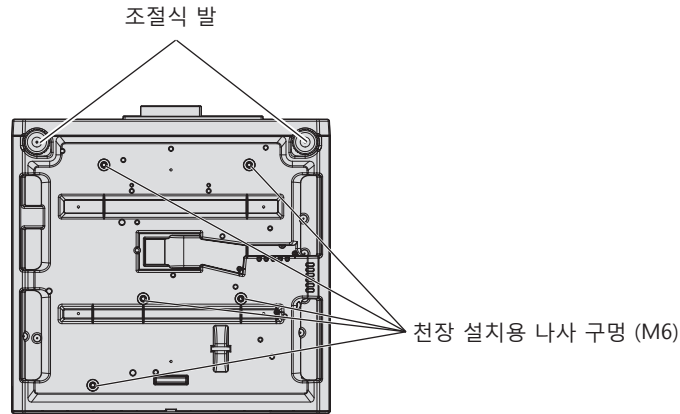
천장 설치용 나사 구멍과 조절식 발의 위치
