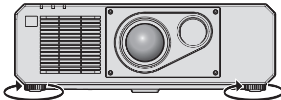
최대 조절 가능 범위 조절식 발: 각각 35 mm (1-3/8")
