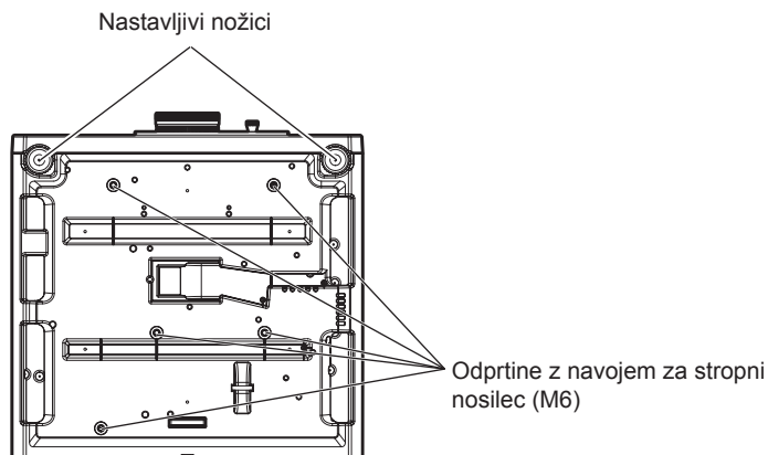
Lega odprtín z navojem za stropni nosilec in nastavljive nožice
