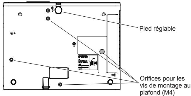
Positions des trous de vis pour le montage au plafond et pied réglable
