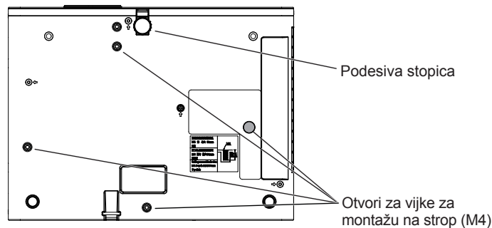
Položaji vijčanih otvora za stropnu montažu i podesivu stopicu
