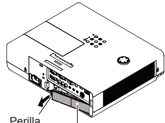
Perilla Unidades de filtro de aire (Trasero)
