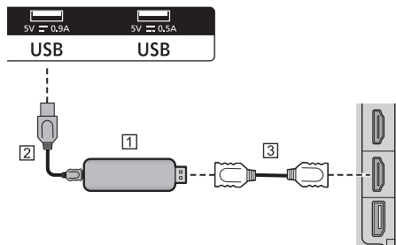
1 Stick PC (disponibile in commercio)
