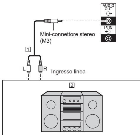
1 Cavo audio stereo (disponibile in commercio)
