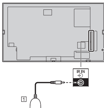
1 Sensore IR (accessorio in dotazione)
